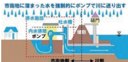
排水機場の仕組み
