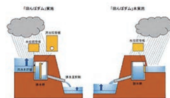
「田んぼダム」を実施している 水田の排水イメージ
