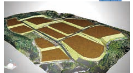
実施設計の3次元化(ICT工事にも活用)
